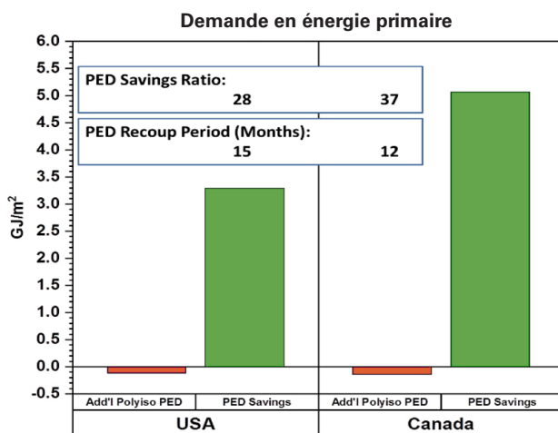
Illustration 5 Résultats de la moyenne nationale quant à la demande en énergie primaire
